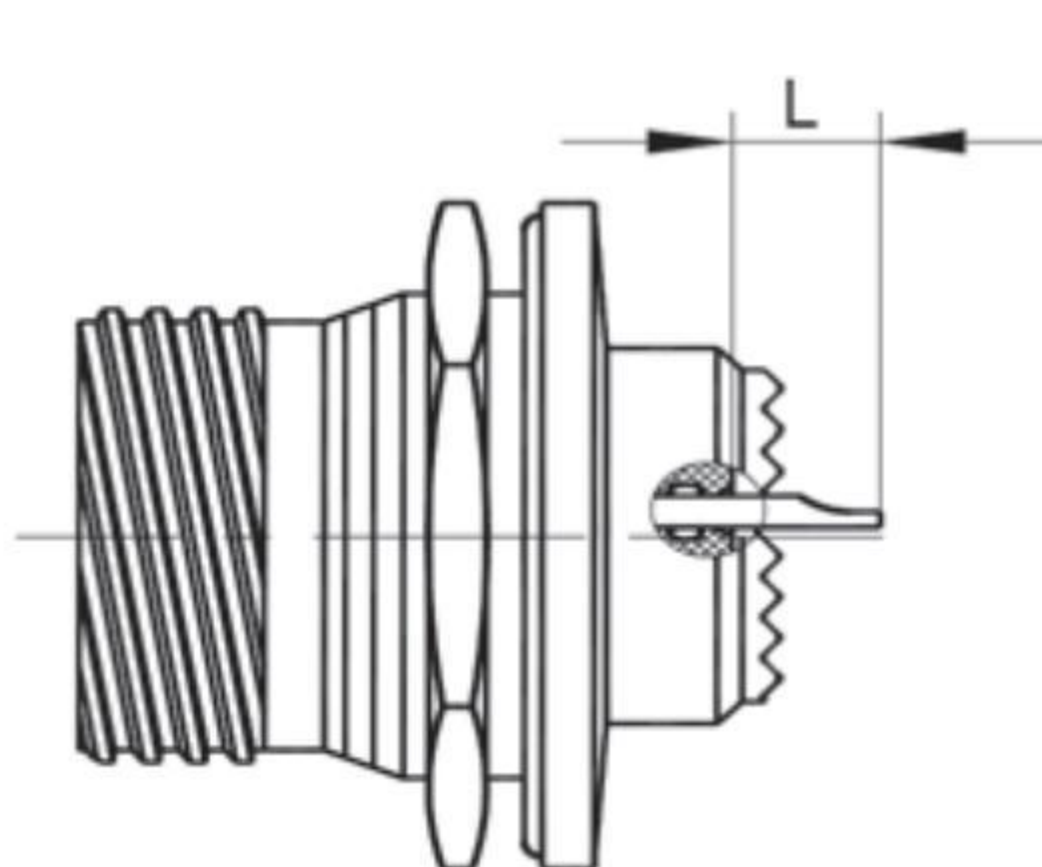
24 Type Receptacle
