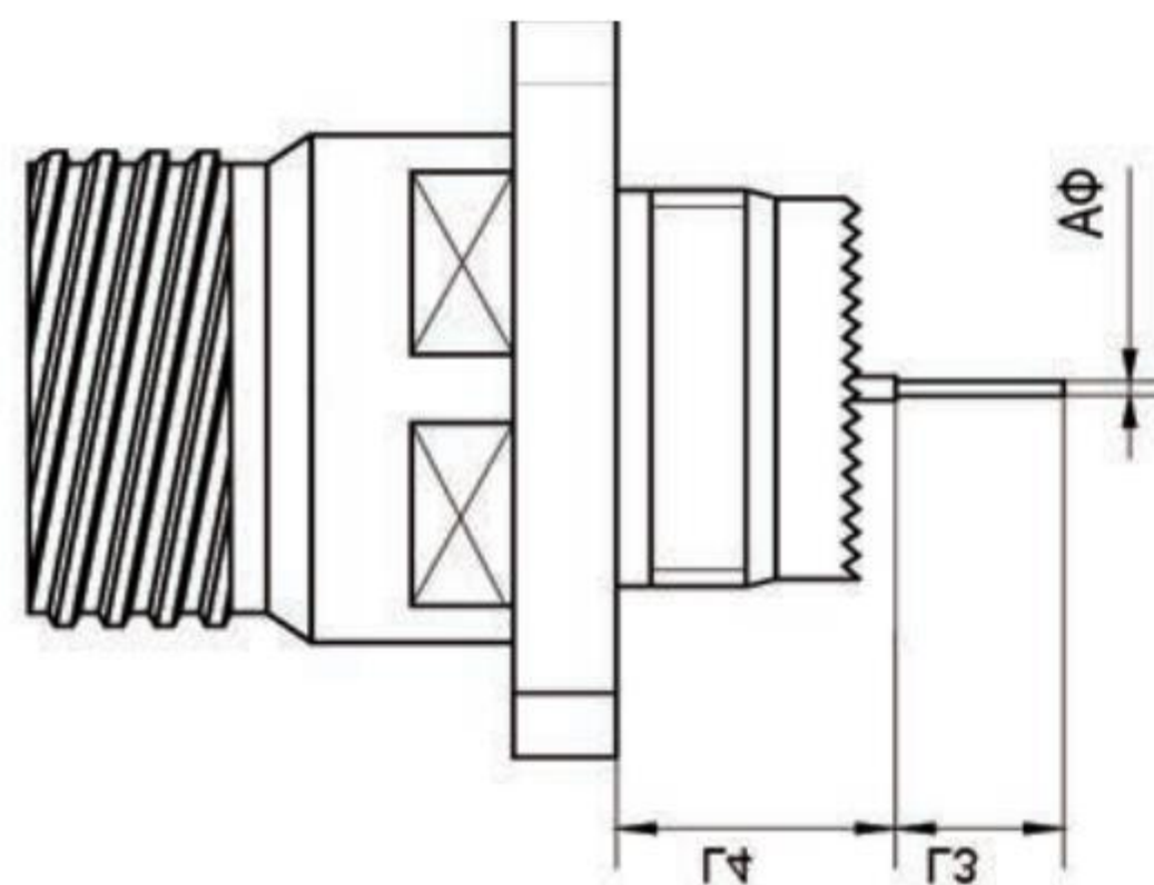
38999/20 Type Receptacle
