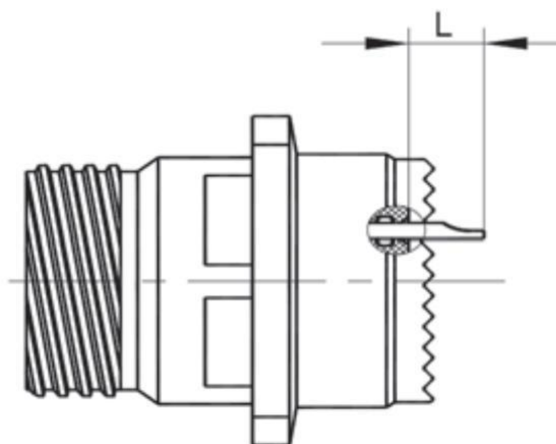
20 Type Receptacle
